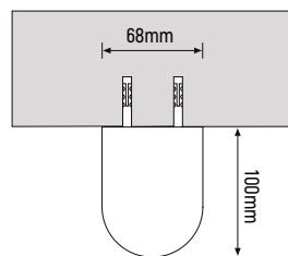
Montaggio a soffitto
