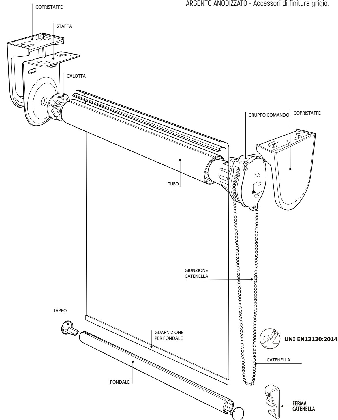
Montaggio a soffitto
