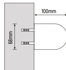
Montaggio a parete
